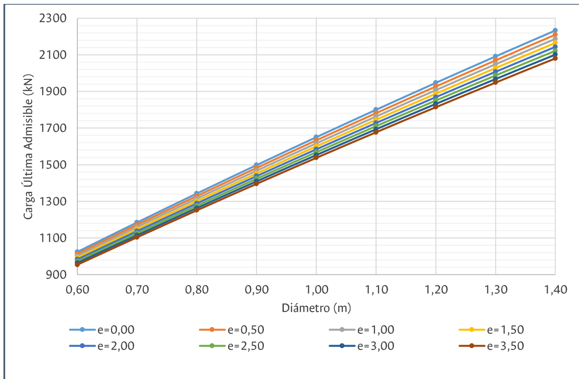
Figura 5. Capacidad lateral de pilotes individuales de 57 m de longitud. Valores en kN
