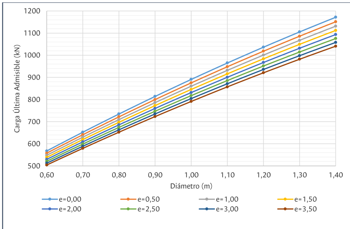
Figura 2. Capacidad lateral de pilotes individuales de 35 m de longitud. Valores en kN
