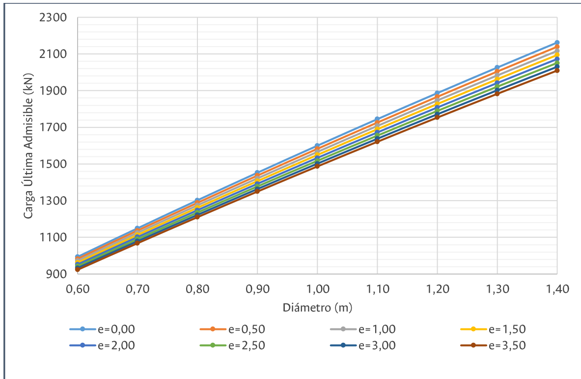
Figura 4. Capacidad lateral de pilotes individuales de 56 m de longitud. Valores en kN
