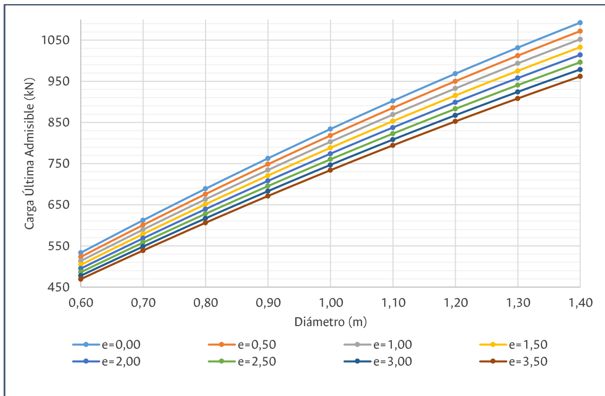
Figura 1. Capacidad lateral de pilotes individuales de 33 m de longitud. Valores en kN
