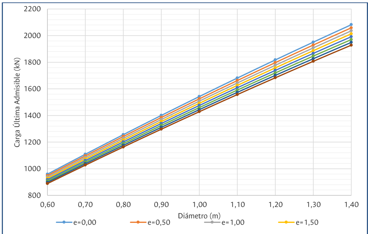
Figura 3. Capacidad lateral de pilotes individuales de 55 m de longitud. Valores en kN
